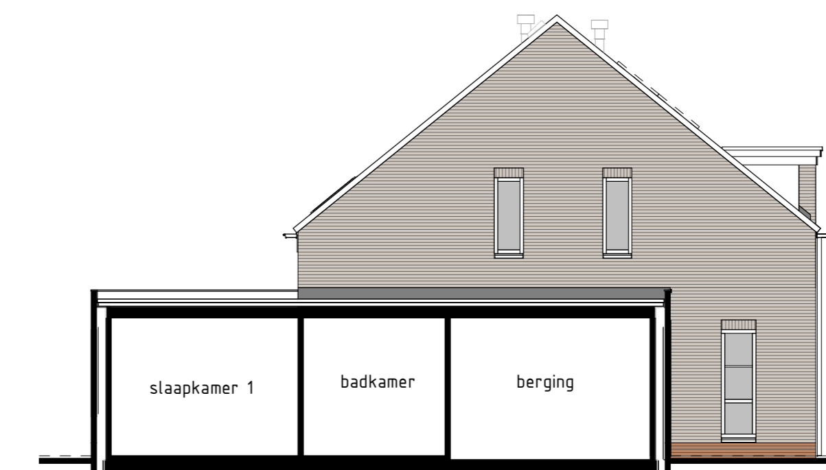
type F3 bwnr get.:218 LINKER ZIJGEVEL
