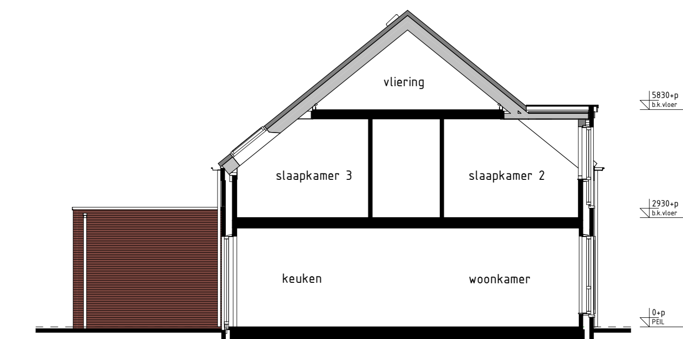
type F1, F1sp, F2sp, F3 bwnr get.:216, 218 bwnr gesp.:217, 219 DOORSNEDE F1-F1
