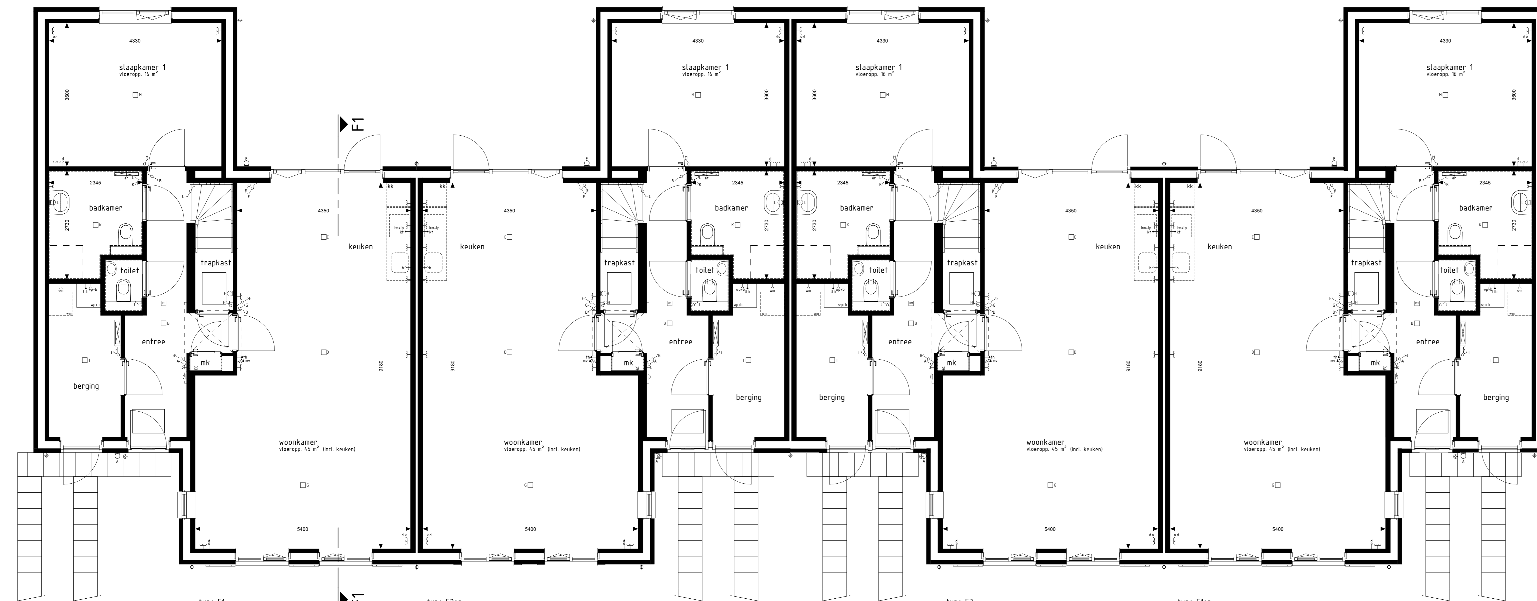
type F1 bwnr get.:216 type F2sp bwnr get.:217 type F3 bwnr get.:218 type F1sp bwnr get.:219 BEGANE GROND
